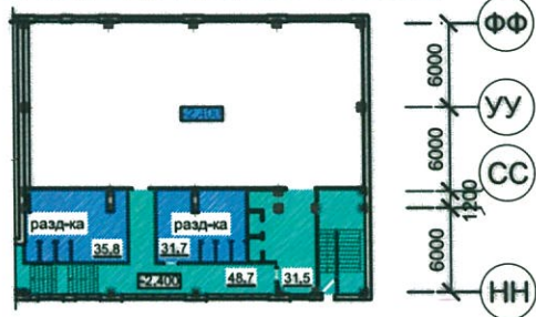
ФРАГМЕНТ ПЛАНА СПОРТЗАЛА НА ОТМ. -2.400
